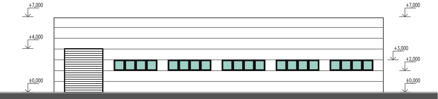
POHL'AD SEVERNÝ
